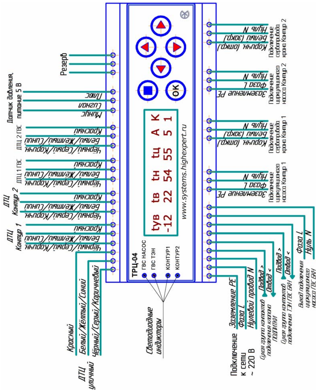
Фигура 1. Схема подключения нагрузок и термдатчиков ДТЦ к контроллеру TRC-04
